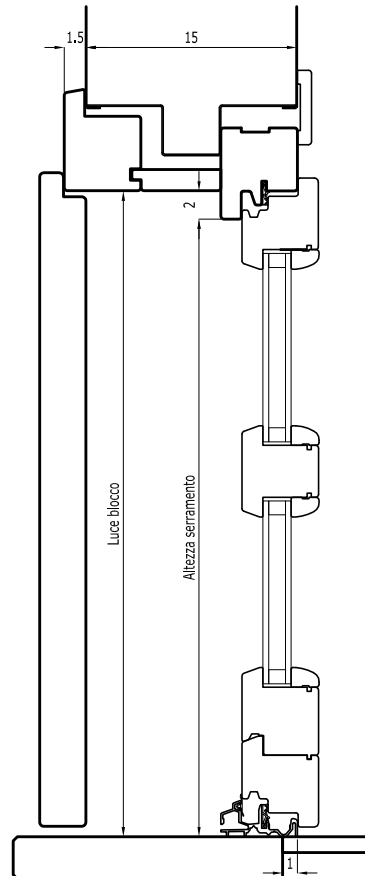
Sezione verticale portafinestra
