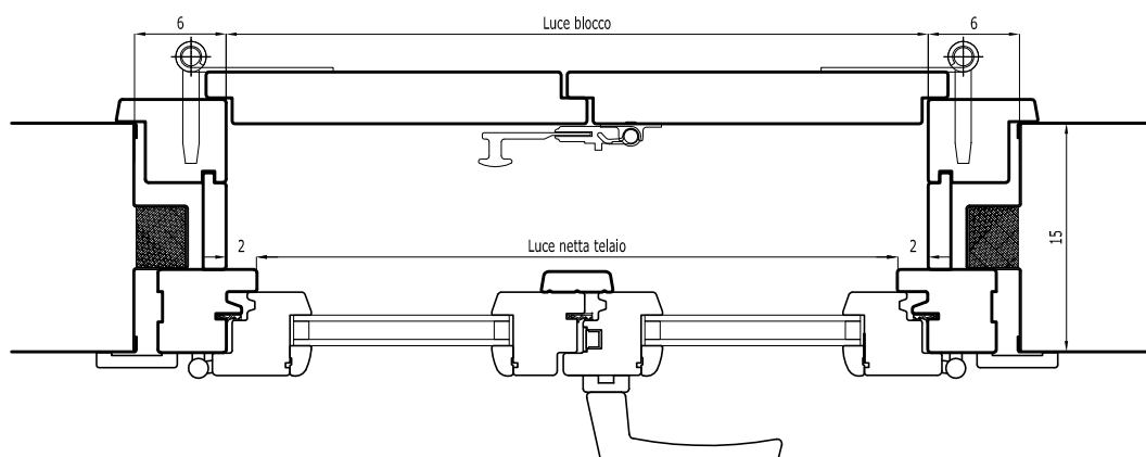
Sezione orizzontale
