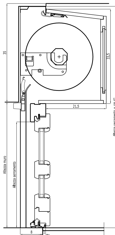
Sezione verticale portafinestra
