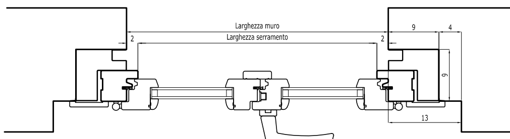
Sezione orizzontale
