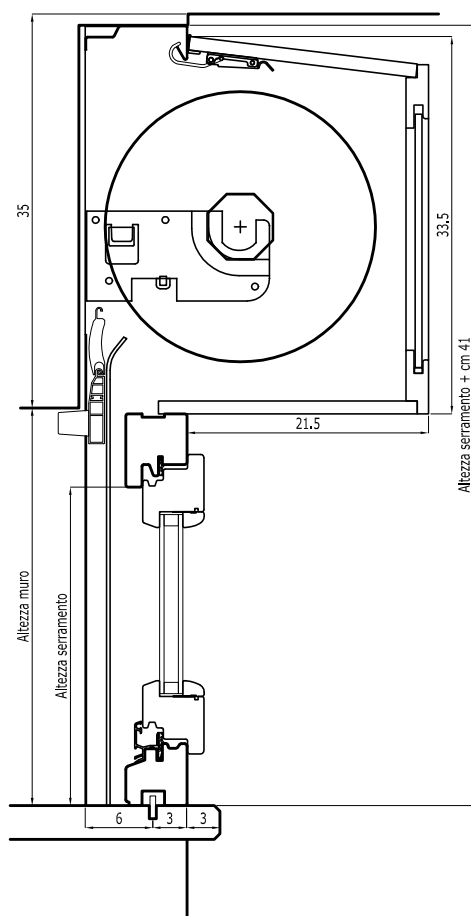
Sezione verticale finestra
