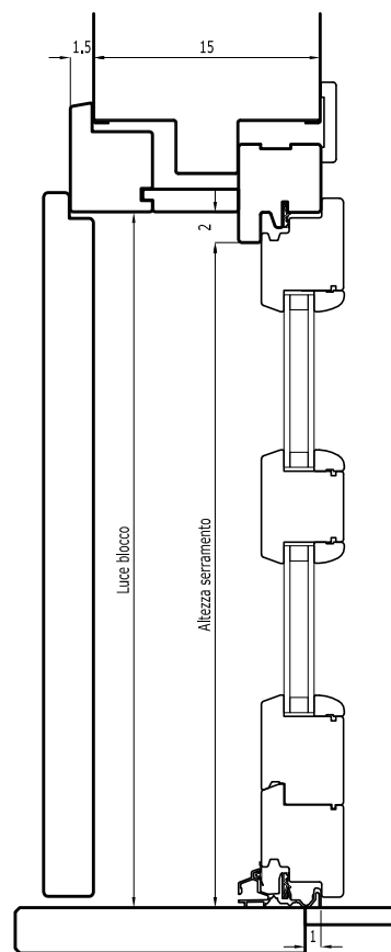
Sezione verticale portafinestra
