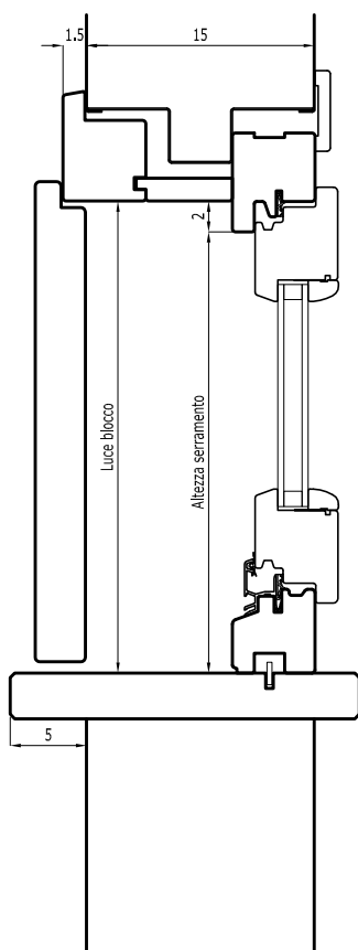
Sezione verticale finestra
