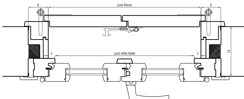
Sezione orizzontale
