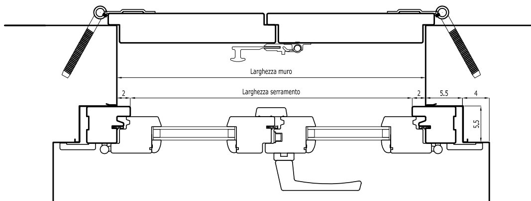
Sezione orizzontale
