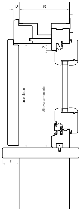
Sezione verticale finestra
