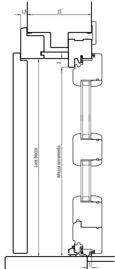
Sezione verticale portafinestra
