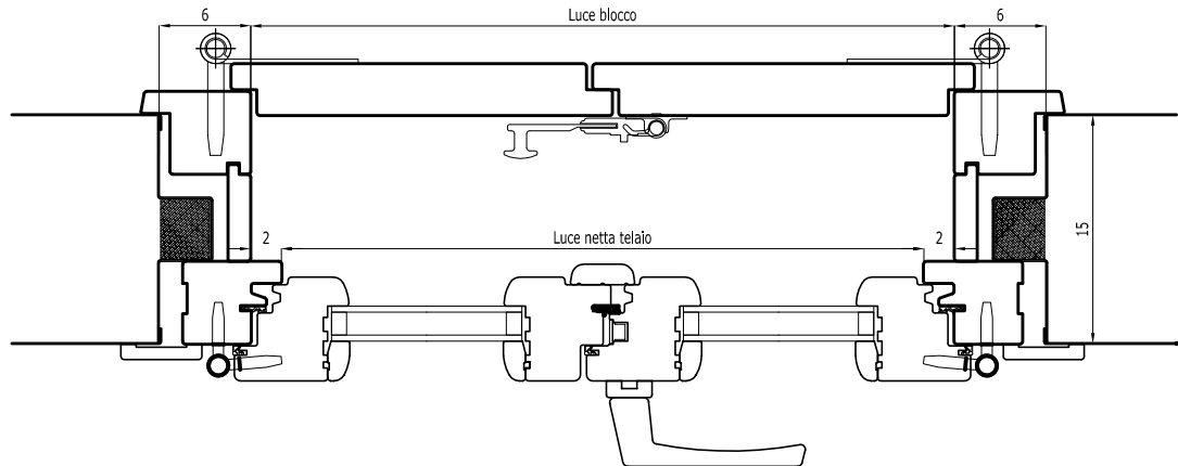
Sezione orizzontale
