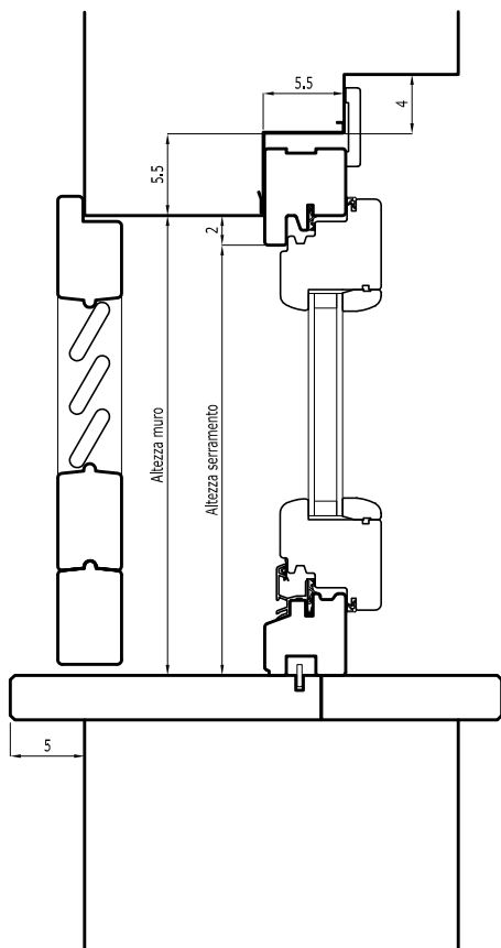
Sezione verticale finestra
