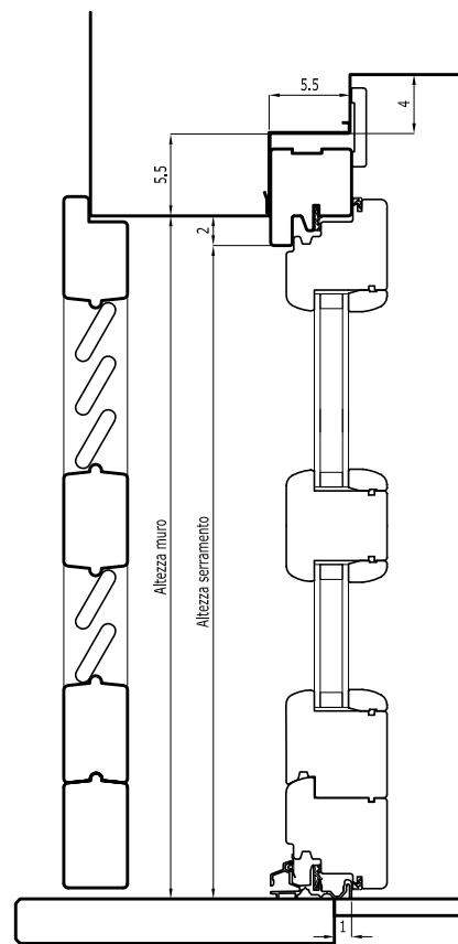
Sezione verticale portafinestra
