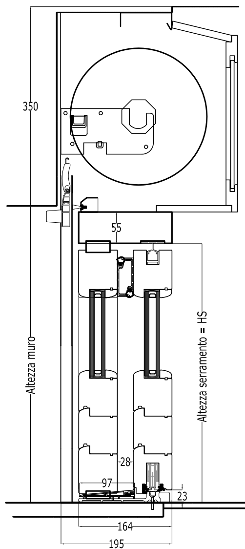
Sezione verticale
