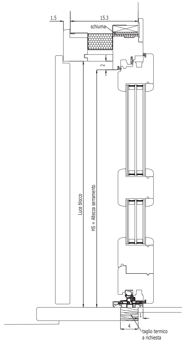
Sezione verticale portafinestra
