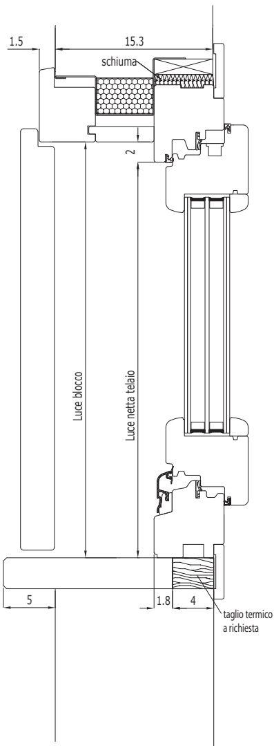
Sezione verticale finestra
