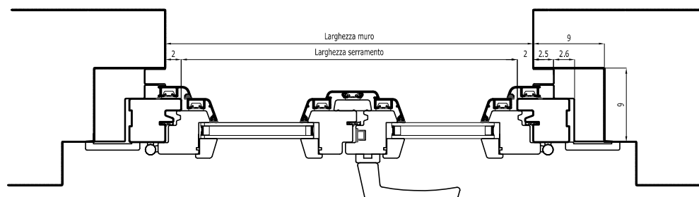
Sezione orizzontale
