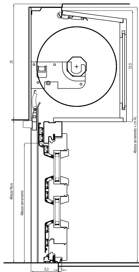
Sezione verticale portafinestra
