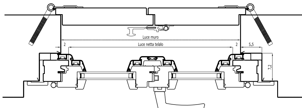
Sezione orizzontale
