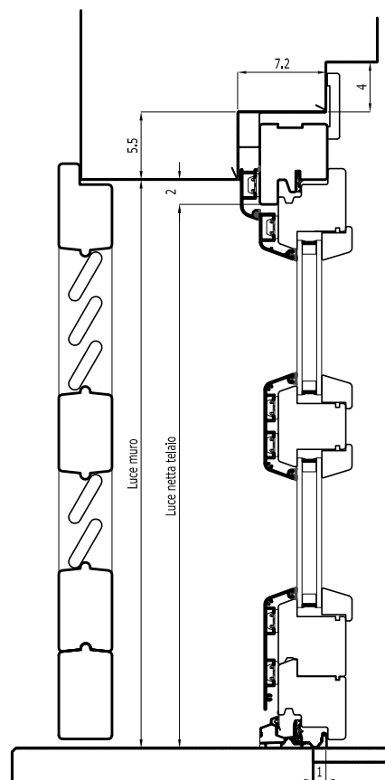
Sezione verticale portafinestra
