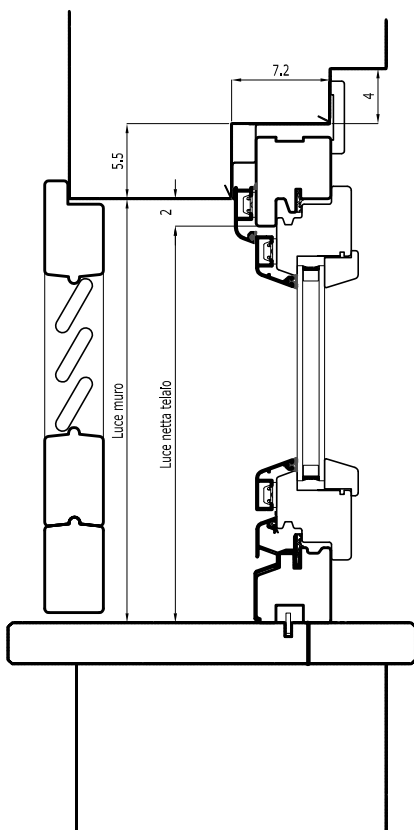
Sezione verticale finestra
