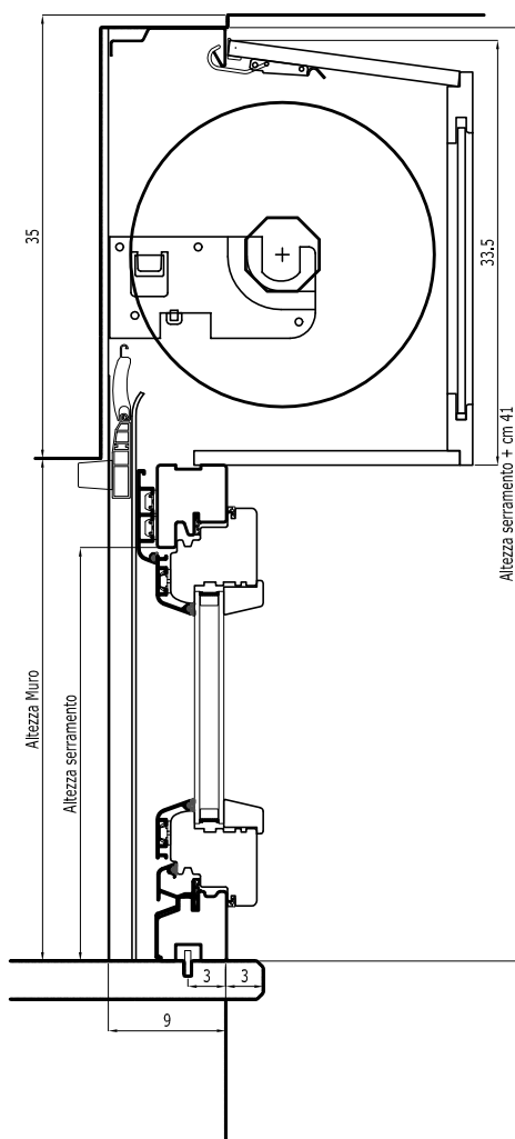
Sezione verticale finestra
