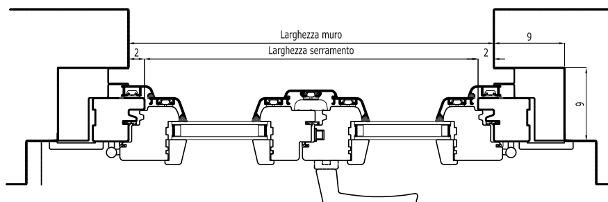
Sezione orizzontale
