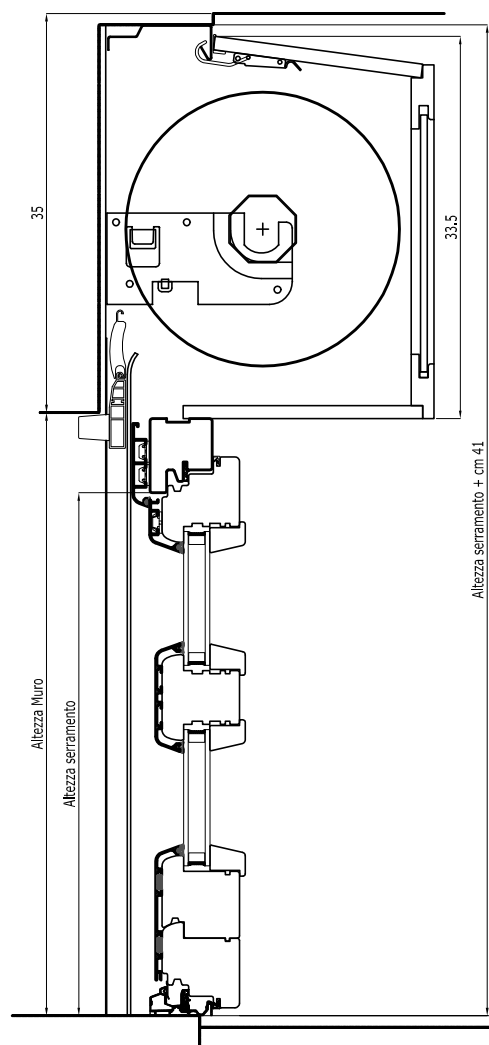
Sezione verticale portafinestra
