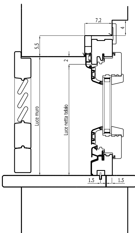
Sezione verticale finestra
