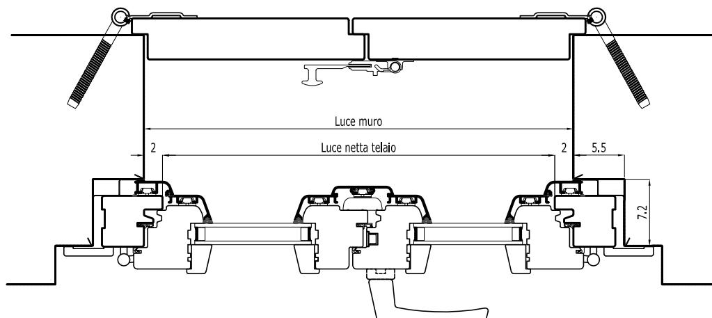
Sezione orizzontale
