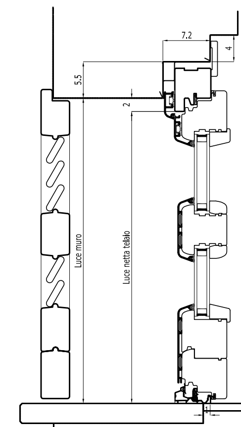
Sezione verticale portafinestra
